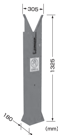
〈外形寸法図〉
