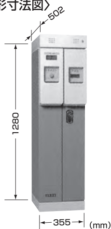
〈外形寸法図〉
