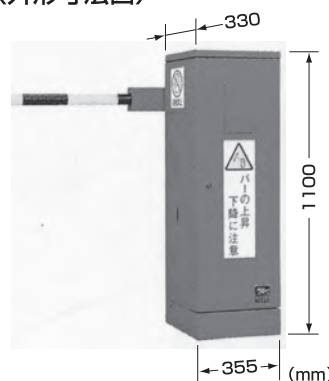
〈外形寸法図〉
